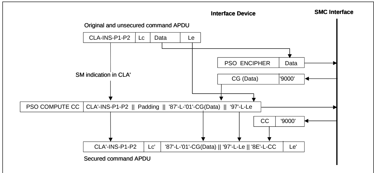
Abbildung 6 – Beispiel der Generierung eines SM-Kommandos
