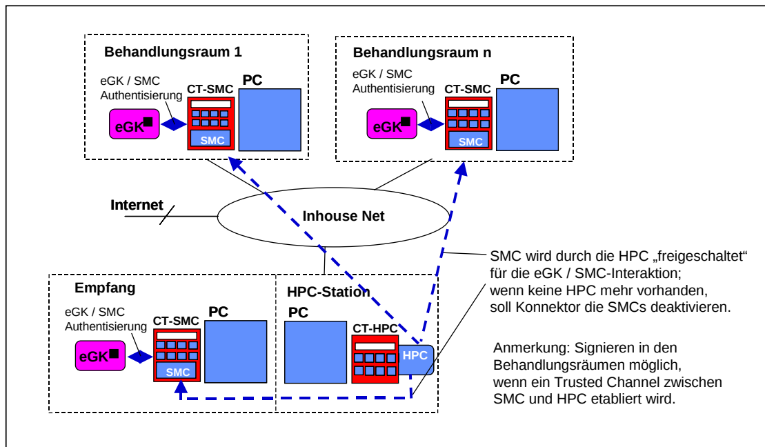
Abbildung 1 - Beispielkonfiguration (vereinfacht) mit logischen Kanälen zur stationären HPC
