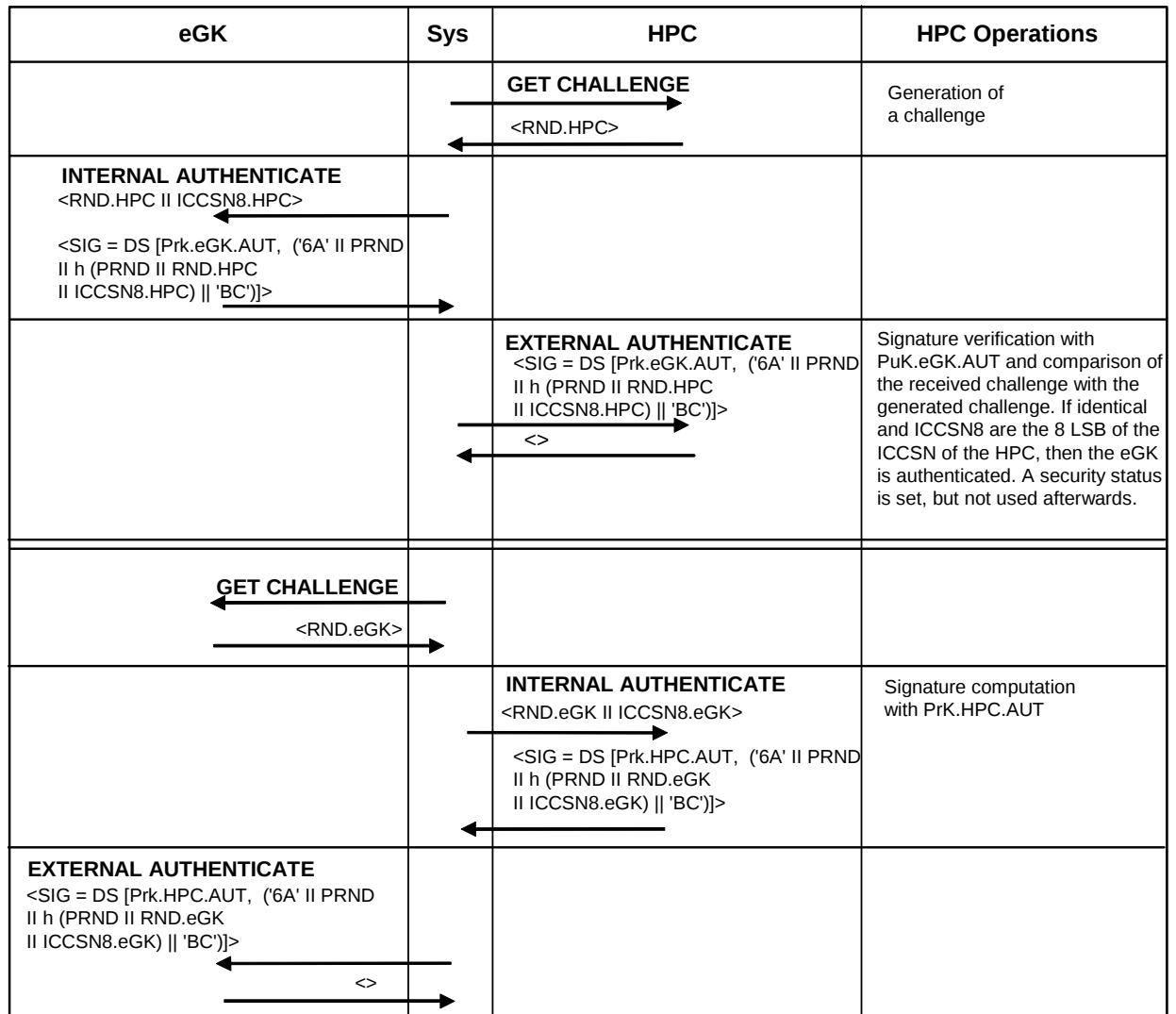
Abbildung 4 – Asymetrisches Authentisierungsverfahren ohne SM-Schlüsselvereinbarung
