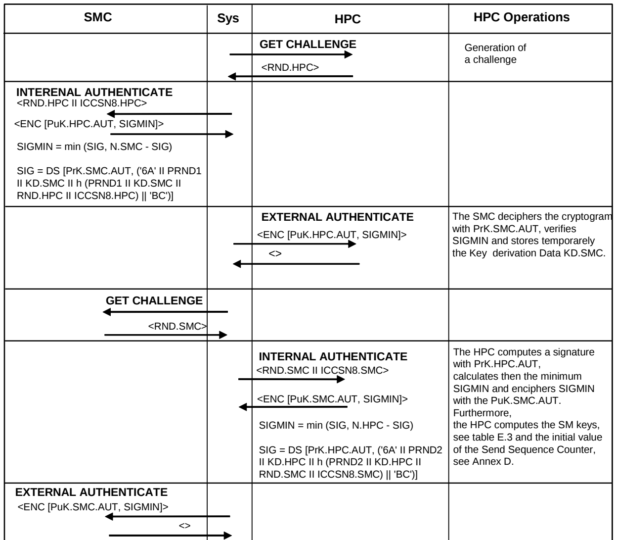
Abbildung 5 – Asymmetrisches Authentisierungsverfahren mit SM-Schlüsselvereinbarung
