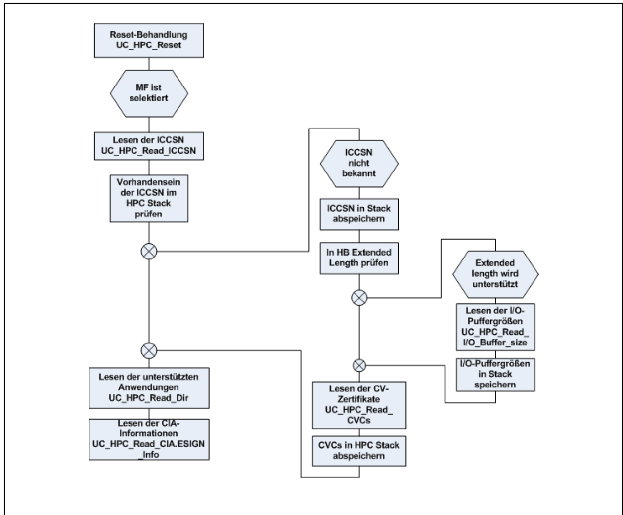
Abbildung 3 – Initialisierungsphase der HPC-Session
