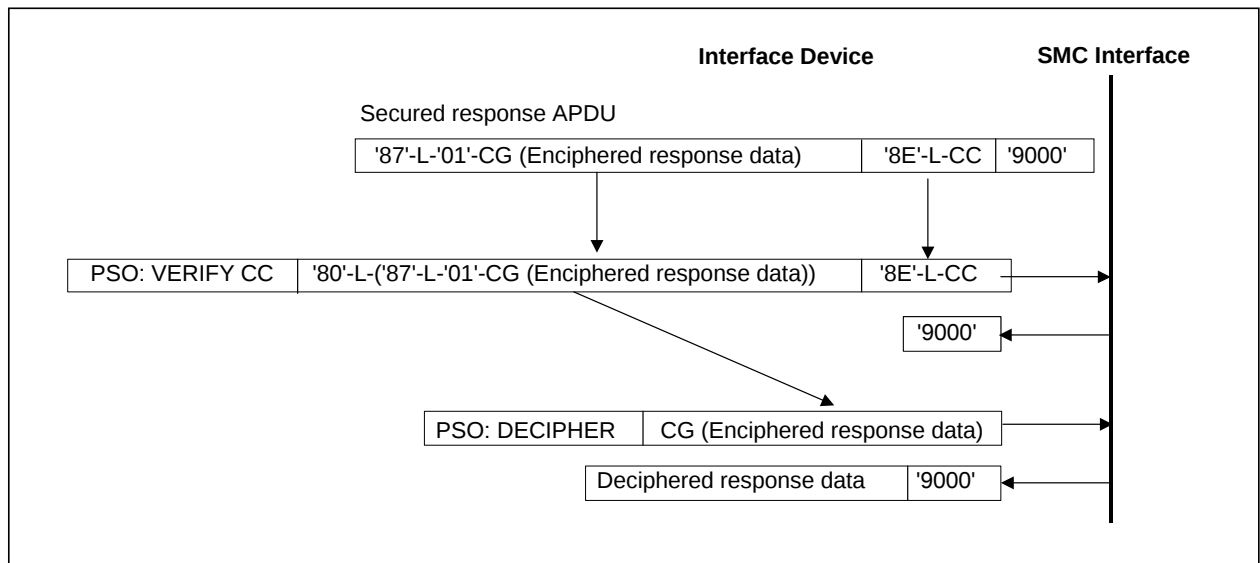
Abbildung 7 – Beispiel der Verarbeitung einer SM-Antwort
